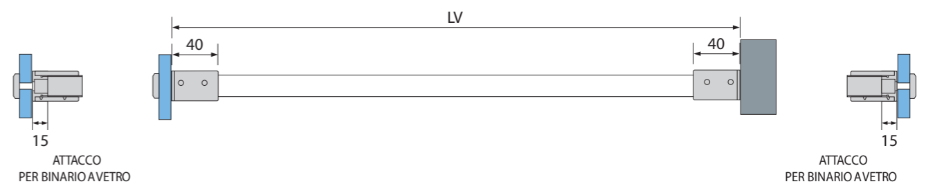
SCHEMA A - PROFILO FERMA ACQUA
