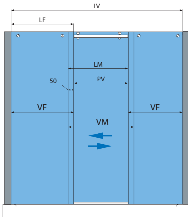
GUIDA PAVIMENTO CON PROFILO FERMA ACQUA
