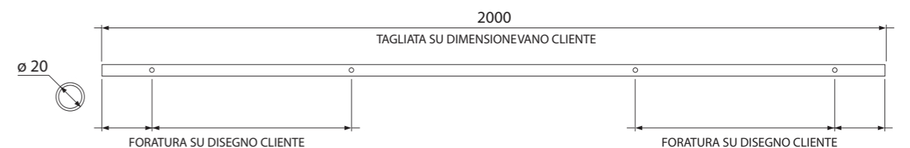
SCHEMA B - BINARIO DI SCORRIMENTO
