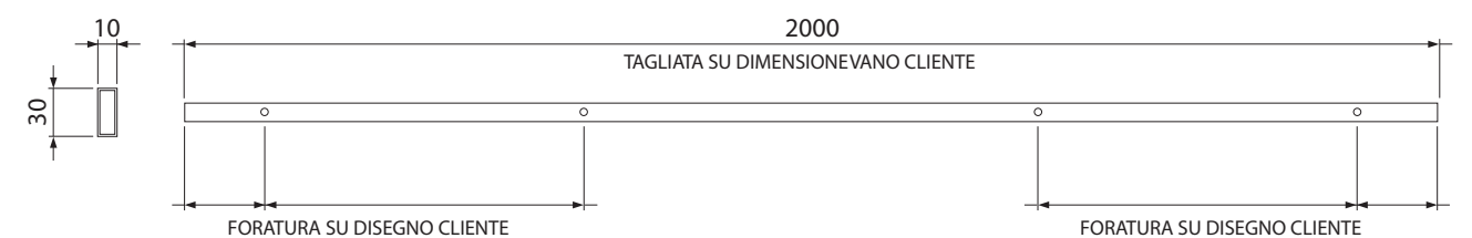
SCHEMA B - BINARIO DI SCORRIMENTO
