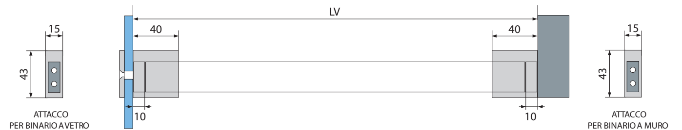
SCHEMA A - PROFILO FERMA ACQUA
