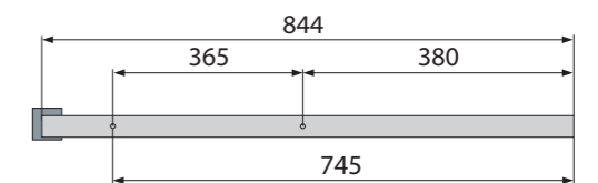
FORATURA DEL BINARIO Piatto doccia 900x900 mm
