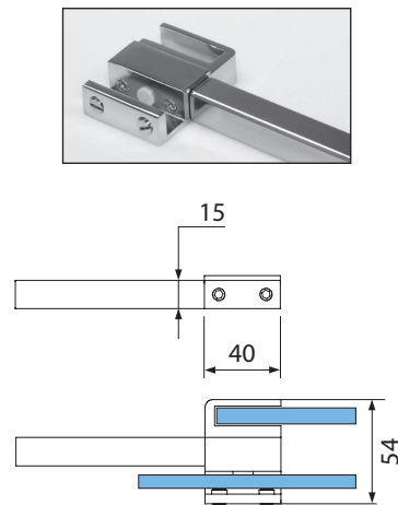
GUIDA PAVIMENTO CON PROFILO FERMA ACQUA
